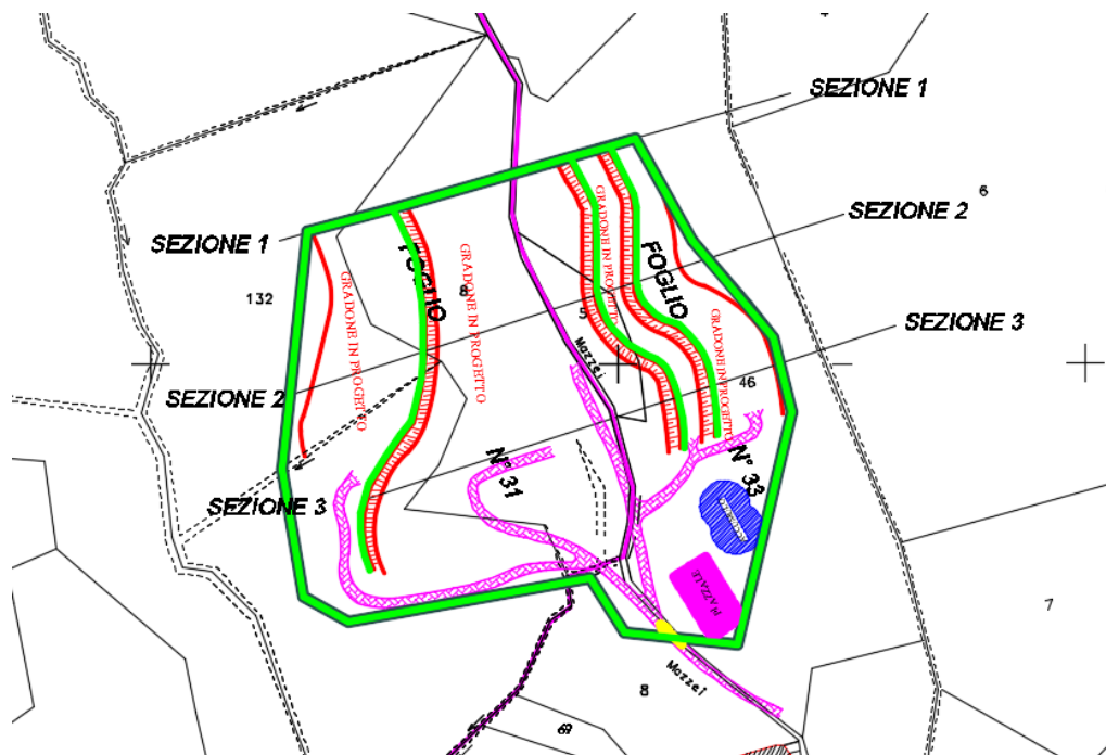
Figura 4.5 – Lay-out gradoni di cava
